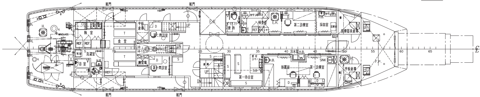
上甲板下
