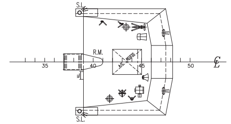
羅針儀甲板
