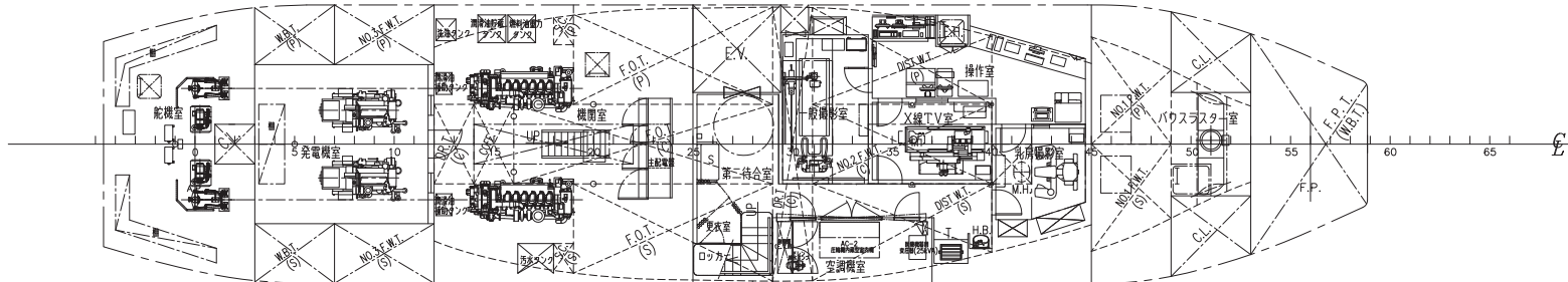
上甲板下
