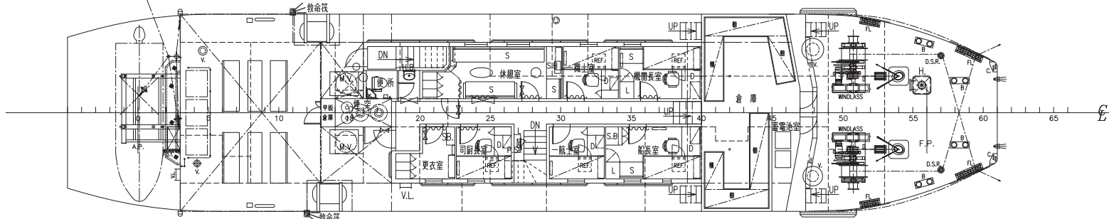
上甲板
